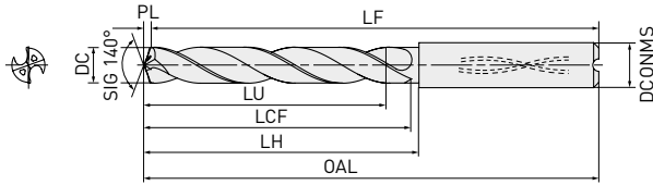
1 Silindirik şaftlı tip
