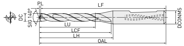
4 Konik boyunlu Whistle notch şaftlı tip
