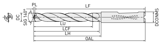
2 Whistle notch şaftlı tip
