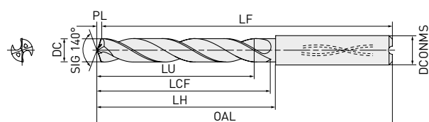
1 Zylind. Schaft
