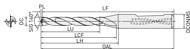
4 Schaft mit Whistle Notch und konischem Hinterschliff
