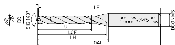
3 Zylind. Schaft mit konischem Hinterschliff
