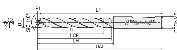
2 Schaft mit Whistle Notch
