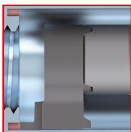
6 TOCZENIE ROWKA CZOŁOWEGO WEWNĘTRZNEGO
