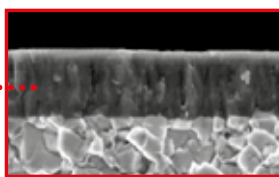
Powłoka PVD na bazie Al-Ti-Cr-N
